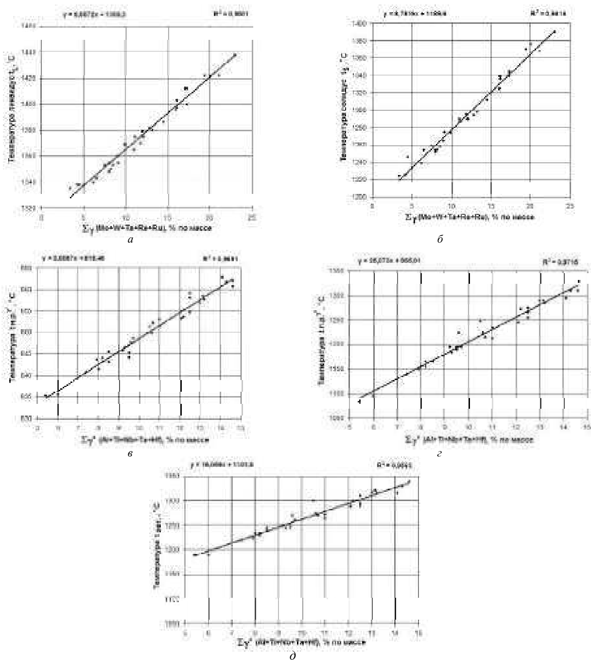
Рис. 3. Математические регрессионные модели для расчета температур t_L , t_S по величине \Sigma C_i^\gamma и температур t_{ЭВТ} , t_{П.Р.} , t_{Н.Р.} по величине \Sigma C_i^\gamma в составе литейных ЖНС
