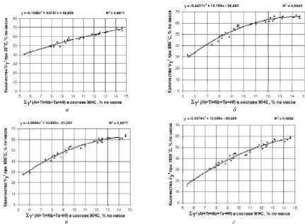
Рис. 5. Математические регрессионные модели для расчета количества V_{\gamma'}^t \gamma' - фазы по суммарному содержанию \Sigma C_i^{\gamma'} \gamma' - образующих элементов в составе ЖНС: а – 20 °С; б – 800 °С; в – 900 °С; г – 1000 °С
