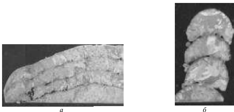
Рис. 6. Макроструктура полученных образцов: а – продольный шлиф, б – поперечный шлиф
