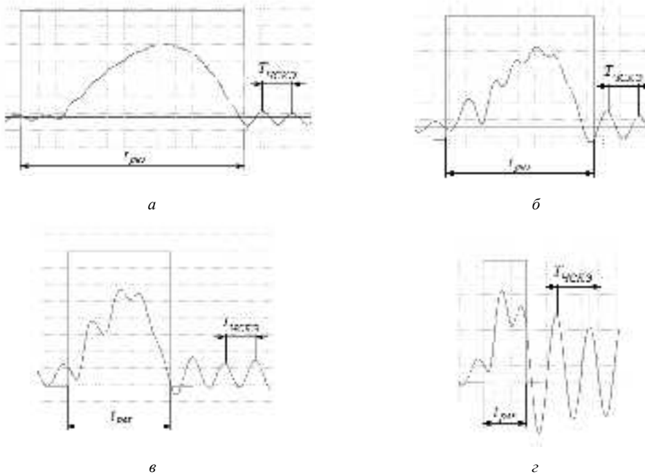
Рис. 14. Фрагменты осциллограмм колебательного движения ТЭ детали:
