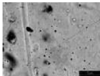
Рис. 8. Топография поверхности покрытия ПГ-СР4 после обработки МЭШ с режимом, указанным в табл. 6 ( \times 200 )
