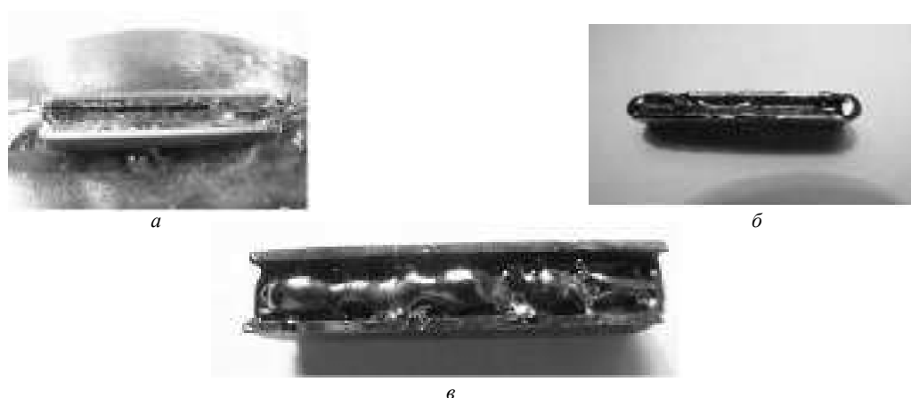
Рис. 1. Внешний вид опытных образцов, полученных с использованием порошка марки BT1-0 (фракция -0,63/+0,315 мм):
