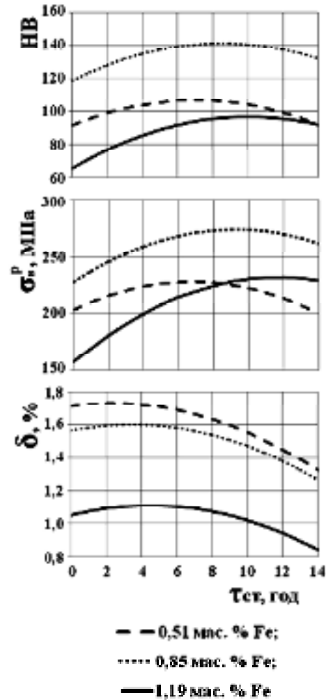
Рис. 2. Залежність механічних властивостей силуміну АК8МЗ від часу витримки при старінні ( \tau_T = 6 год)
