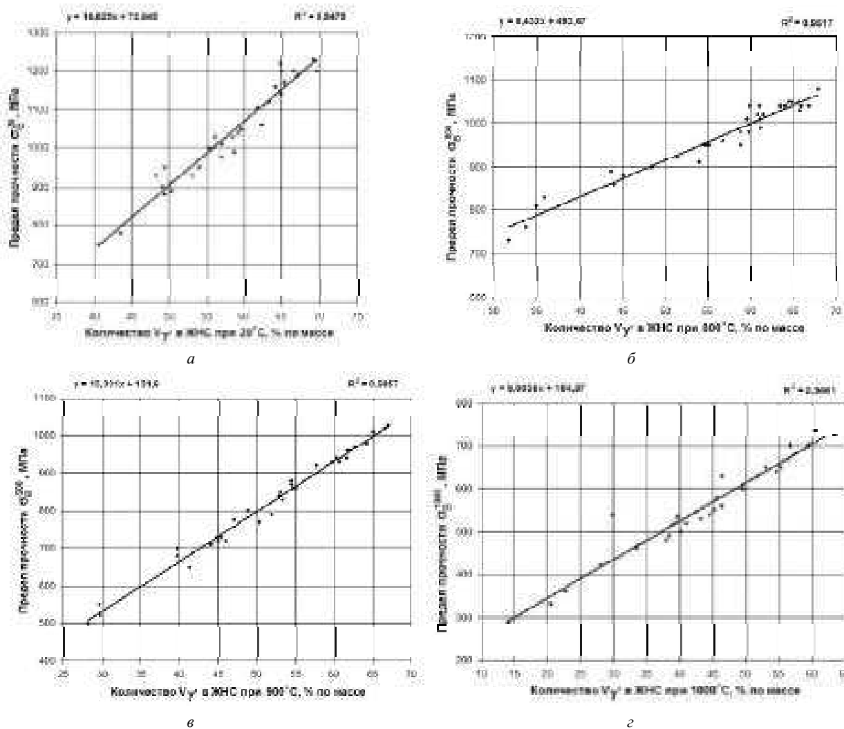
Рис. 6. Математические регрессионные модели для расчета предела кратковременной прочности \sigma_B^t по количеству \gamma' - фазы V_{\gamma'} в литейных ЖНС: а – 20 °С; б – 800 °С; в – 900 °С; г – 1000 °С
