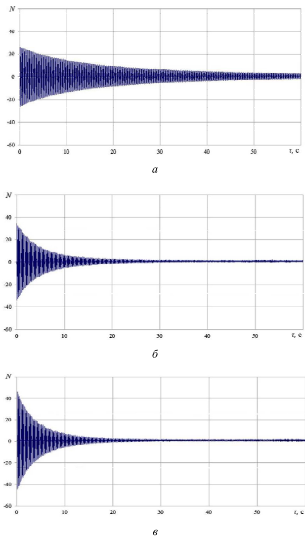
Рис. 1. Віброграми затухаючих коливань зразків зі сталі 20X13:
