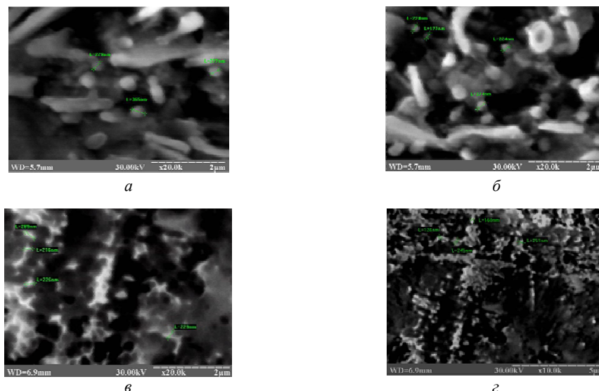
Рис. 2. Мікроструктура сталі 20 після деформації на 48 % (а) і наступної передрекристалізаційної термічної обробки (б) і сталі 20X13 після деформації на 61 % (в) та після передрекристалізаційної термічної обробки (г)
