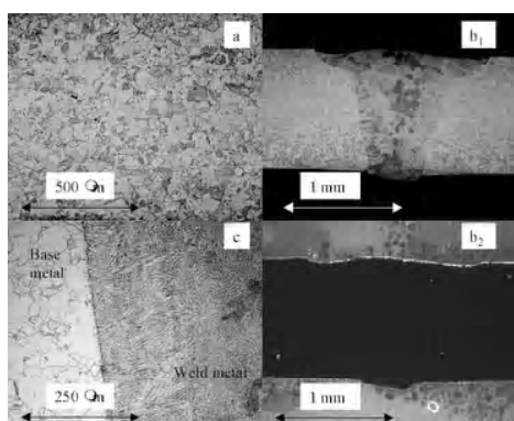
Рис. 4. Микроструктура стали P506 (по С. Сгобба): а – основной металл, в – поперечное сечение сварного шва (в 1 – светлое поле, в 2 – темное поле, травление реактивом Мураками), с – переходная зона от основного к наплавленному металлу
