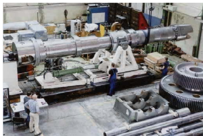
Рис. 6. Шпиндель конструкции фирмы SMS-SIEMAG, позволяющий осевой сдвиг рабочих валков
